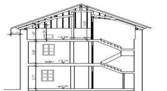
Sección B-B
